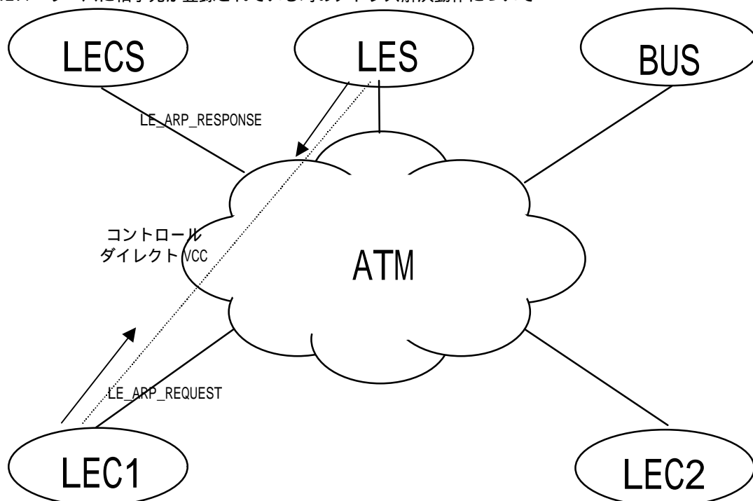
図 3-6 / JF-AF0084.00 補遺 サーバに相手先が登録されている場合の LE_ARP
