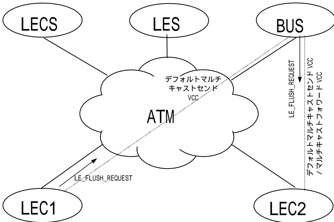
図 4-10 / JF-AF0084.00 補遺 フラッシュ要求の転送の例
