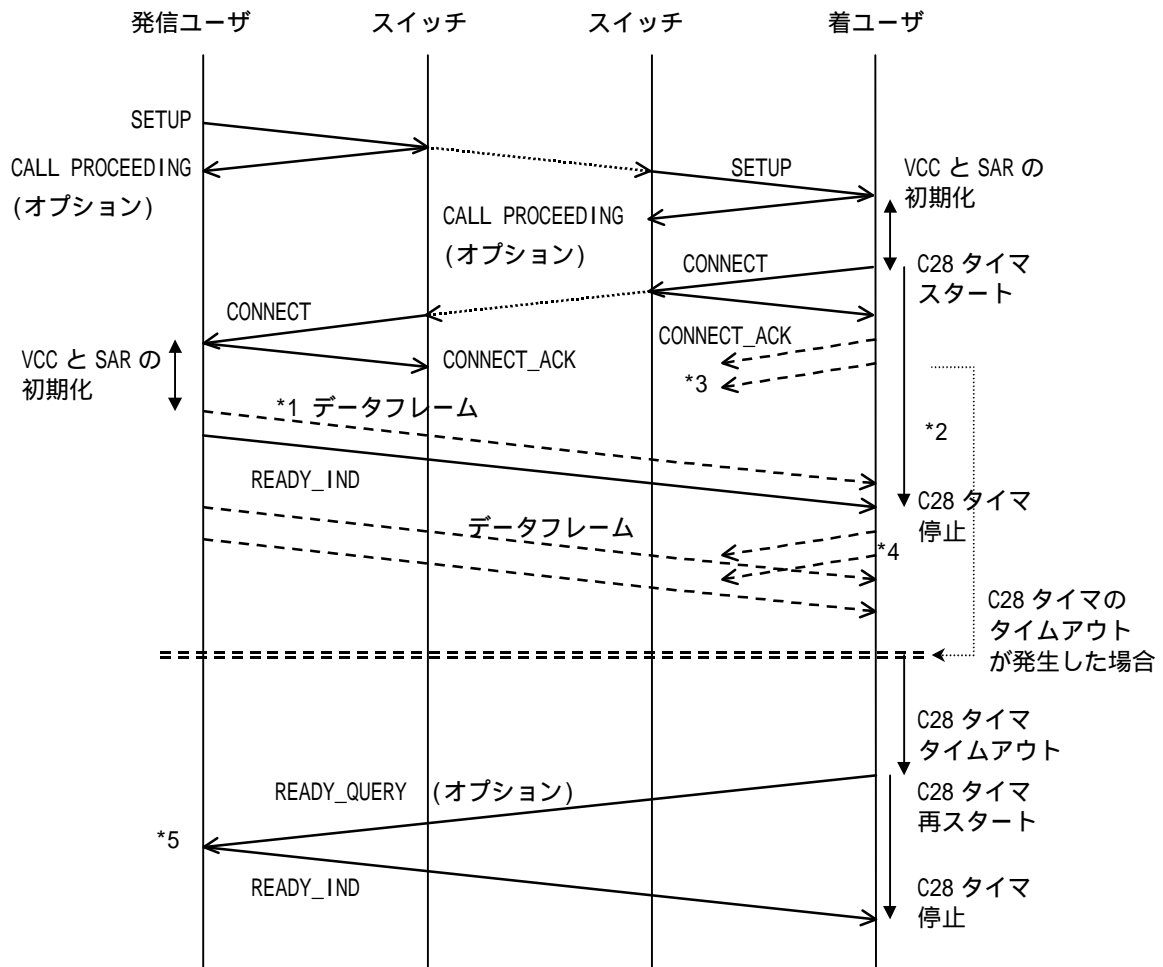
図 3-4 / JF-AF0084.00 補遺 コネクションの確立
