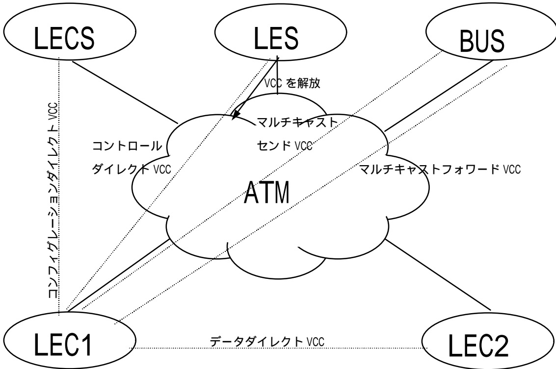
図 4-13 / JF-AF0084.00 補遺 LES からのターミネーションの例
