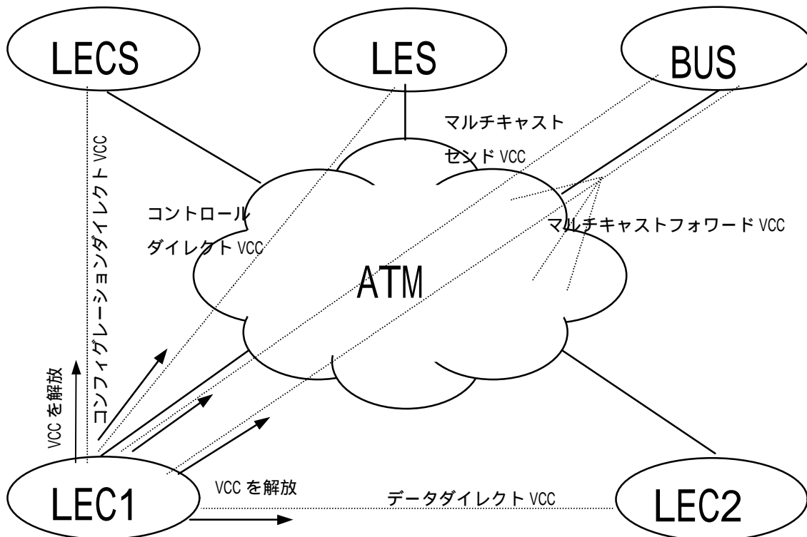
図 4-12 / JF-AF0084.00 補遺 LEC からのターミネーションの例
