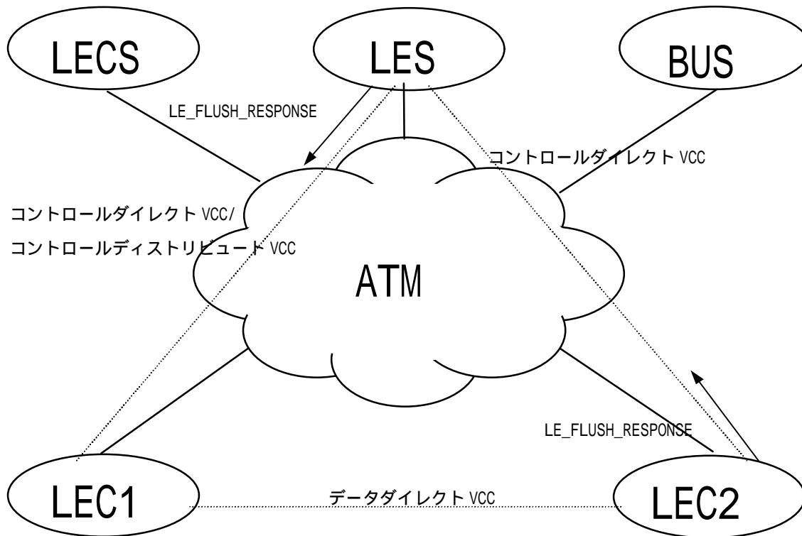
図 4-11 / JF-AF0084.00 補遺 フラッシュ応答の転送の例
