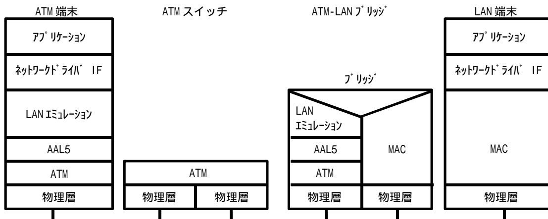
図 1-1 / JF-AF0084.00 補遺 LAN エミュレーションのプロトコルスタック
