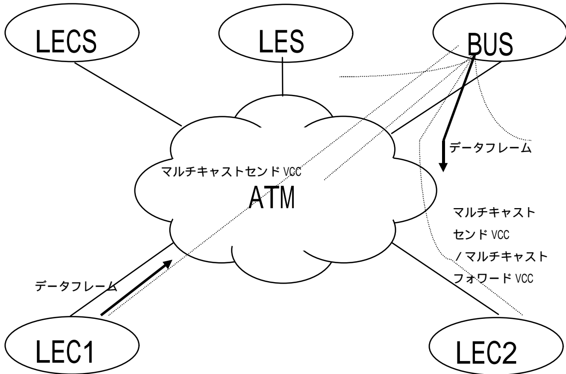
図 4-8 / JF-AF0084.00 補遺 ユニキャストデータ転送 (BUS 経由) の例
