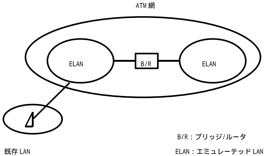
図 1-2 / JF-AF0084.00 補遺 LAN エミュレーションの範囲例
