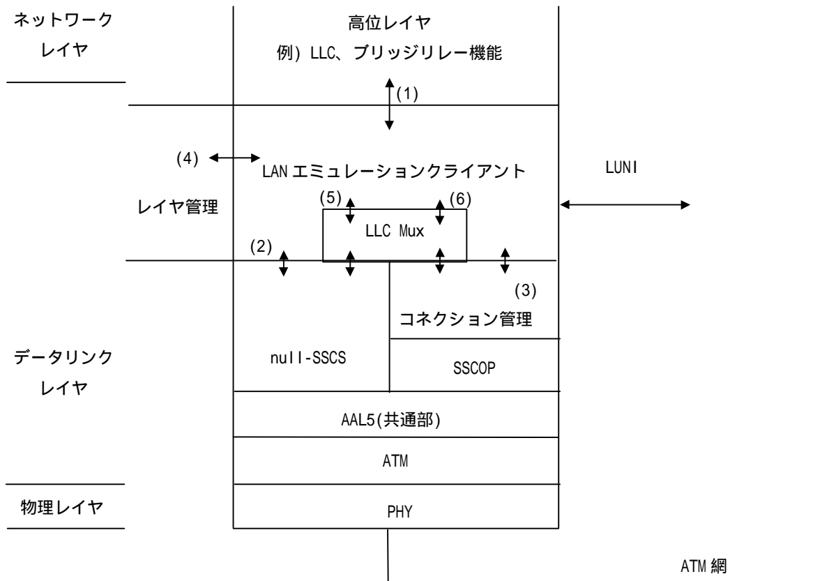
図 3-3 / JF-AF0084.00 補遺 レイヤアーキテクチャに LAN エミュレーションのレイヤアーキテクチャを示す。
