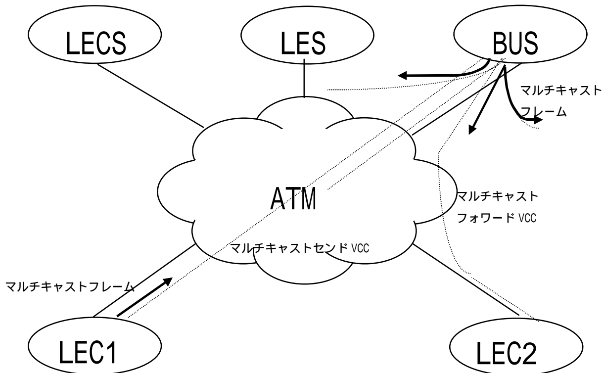
図 4-7 / JF-AF0084.00 補遺 マルチキャストデータ転送の例
