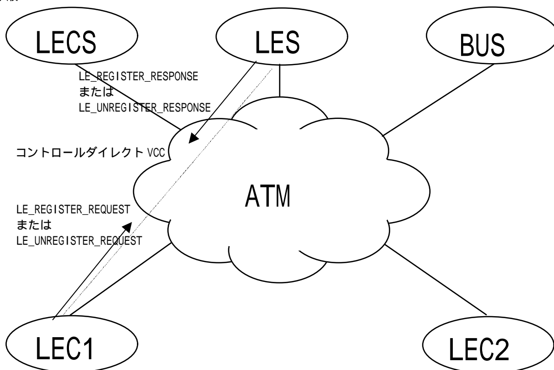
図 4-5 / JF-AF0084.00 補遺 登録の例
