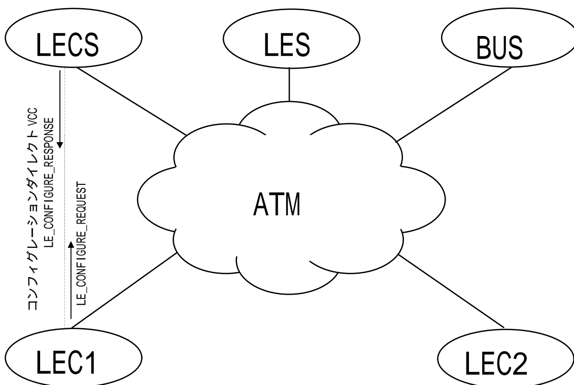
図 4-3 / JF-AF0084.00 補遺 コンフィグレーションフェーズの例
