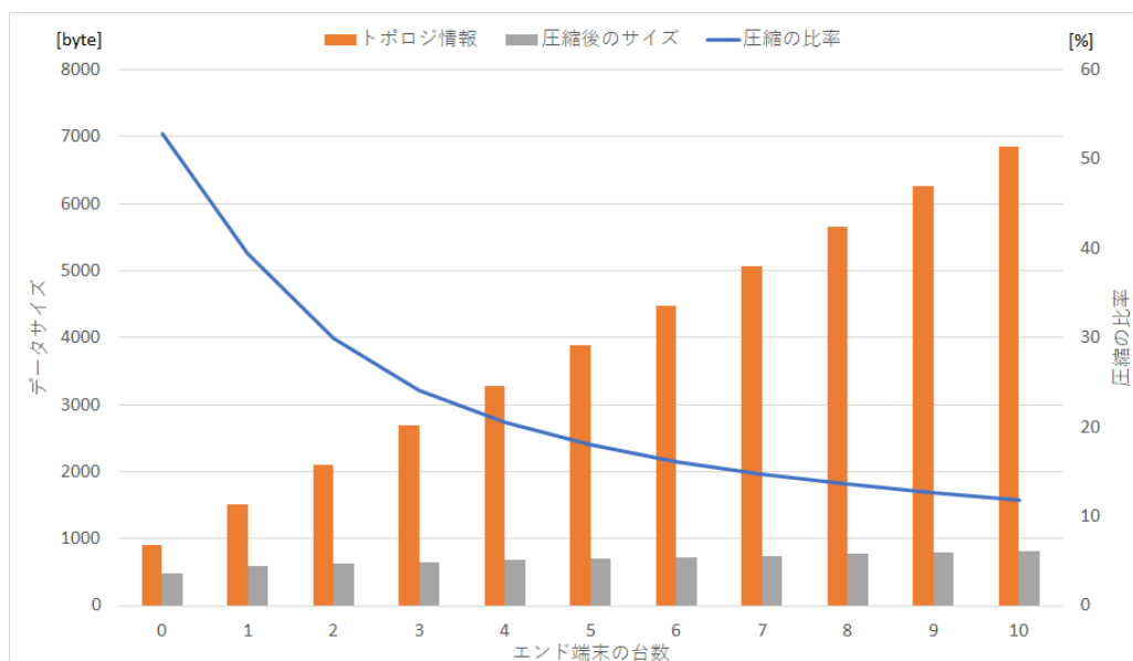
図 8. トポロジ情報の ZIP 圧縮効果
