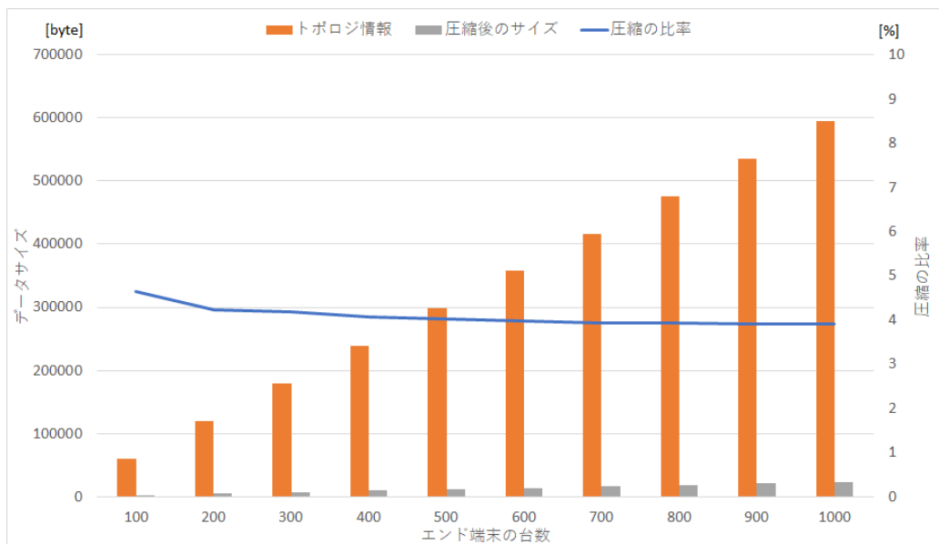
図 C-3. エンド端末数が 100～1,000 台の場合のトポロジ情報・圧縮後のサイズ・圧縮の比率
