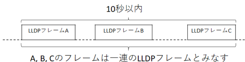
図3. HTIPにおけるLLDPフレーム構成
