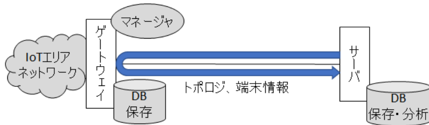
図7. GW-サーバ間通信(サーバ問い合わせ)
