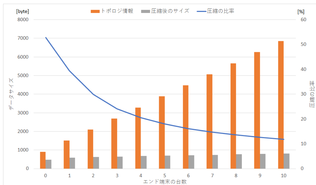
図 C-1. エンド端末数が 0~10 台の場合のトポロジ情報・圧縮後のサイズ・圧縮の比率
