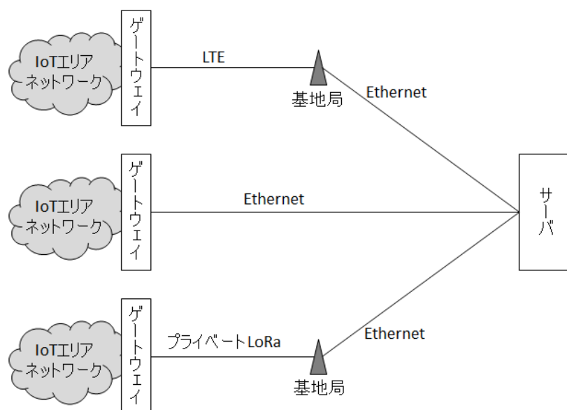
図4. 大規模IoTシステムの構成例
