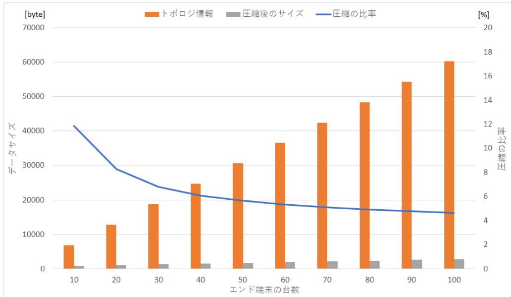
図 C-2. エンド端末数が 10～100 台の場合のトポロジ情報・圧縮後のサイズ・圧縮の比率
