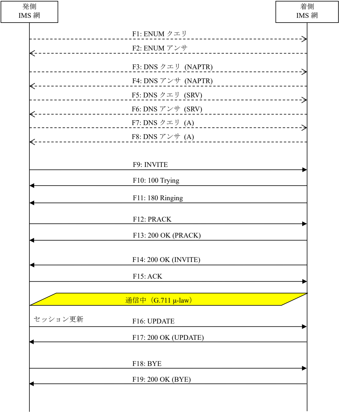
図 4.2.1.1.1-1/TR-1088 発切断- (固定発-固定着 (RBT 送出发側))
