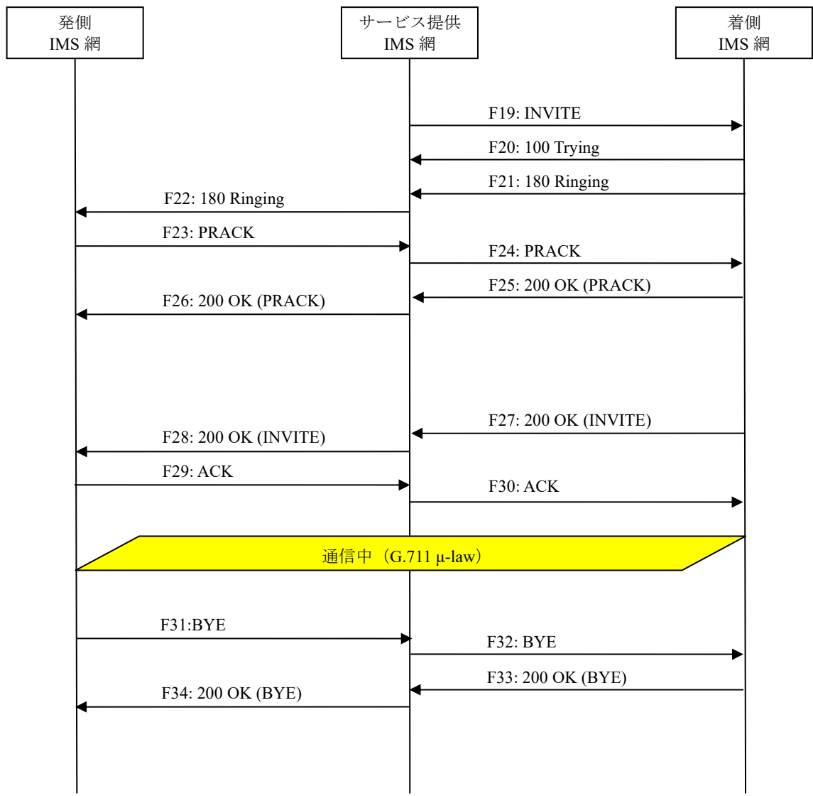
図 4.2.3.4-2／TR-1088 0120/0800/0570 発着接続（転送先特番）（2/2）
