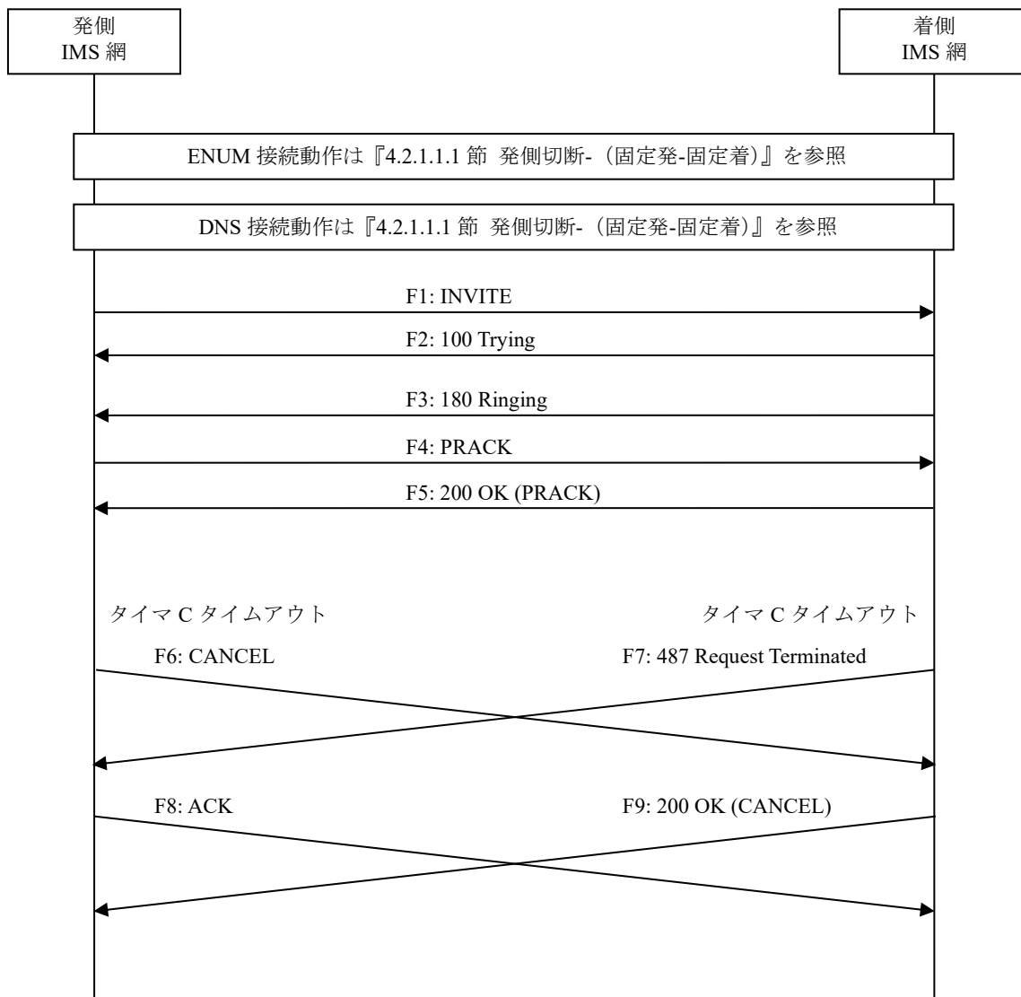
図 4.2.1.2.5-1/TR-1088 途中切断 (タイマ C 満了 発着交差)
