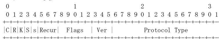
図2-2 LLDPUをカプセル化するGREヘッダのフォーマット
